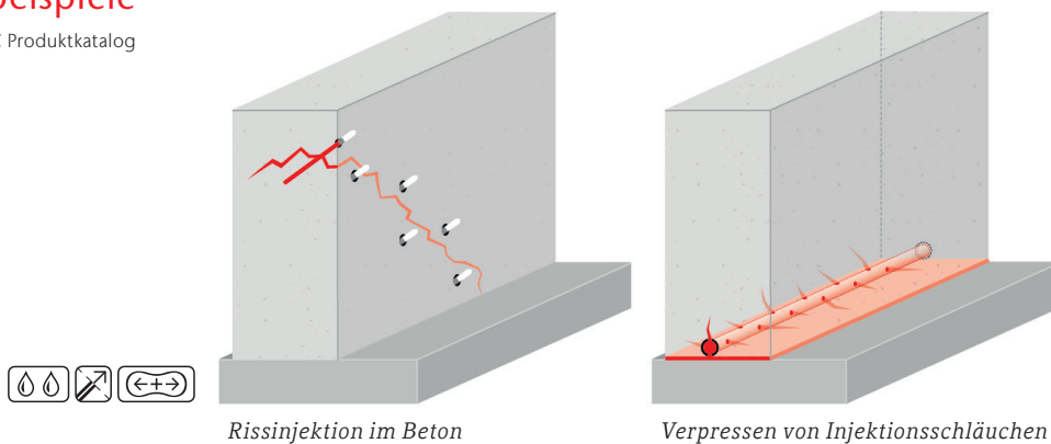
Rissinjektion im Beton
